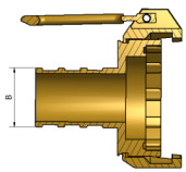
FEMMINA CON MANIGLIA E PORTAGOMMA FEMALE WITH HANDLE AND INSERT
