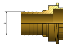
MASCHIO CON PORTAGOMMA MALE WITH INSERT
